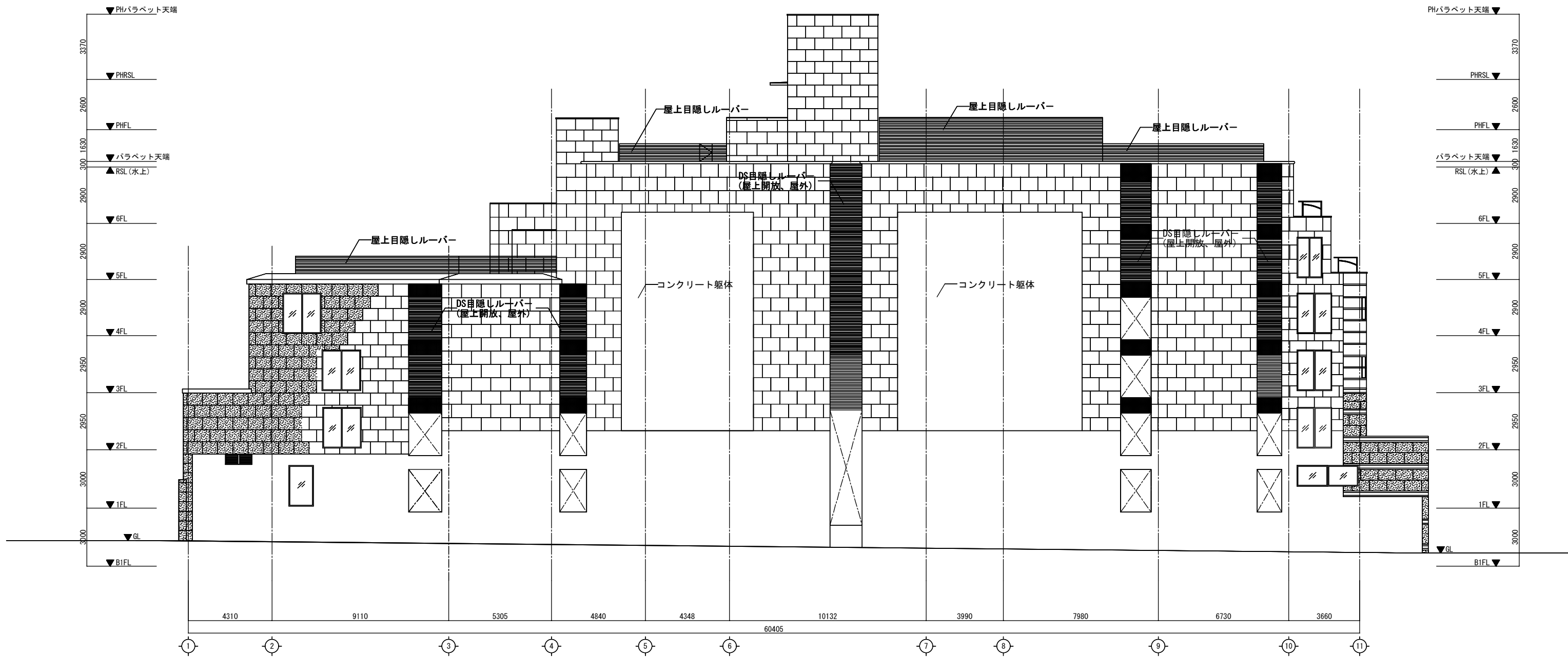
東立面図
