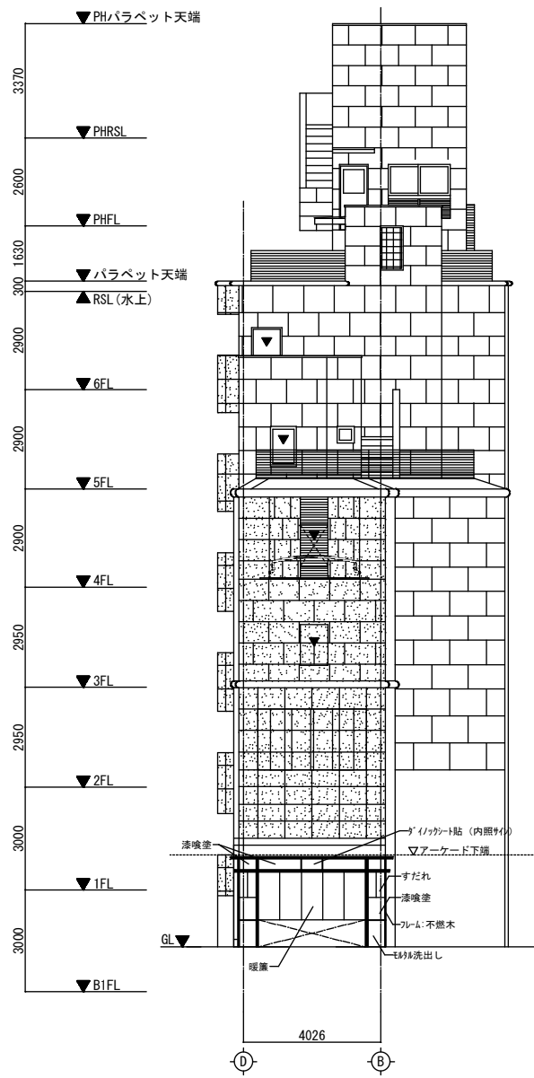
南立面図
