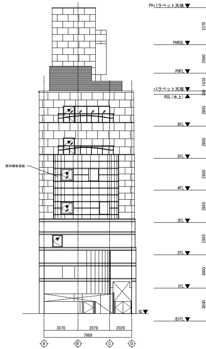
北立面図
