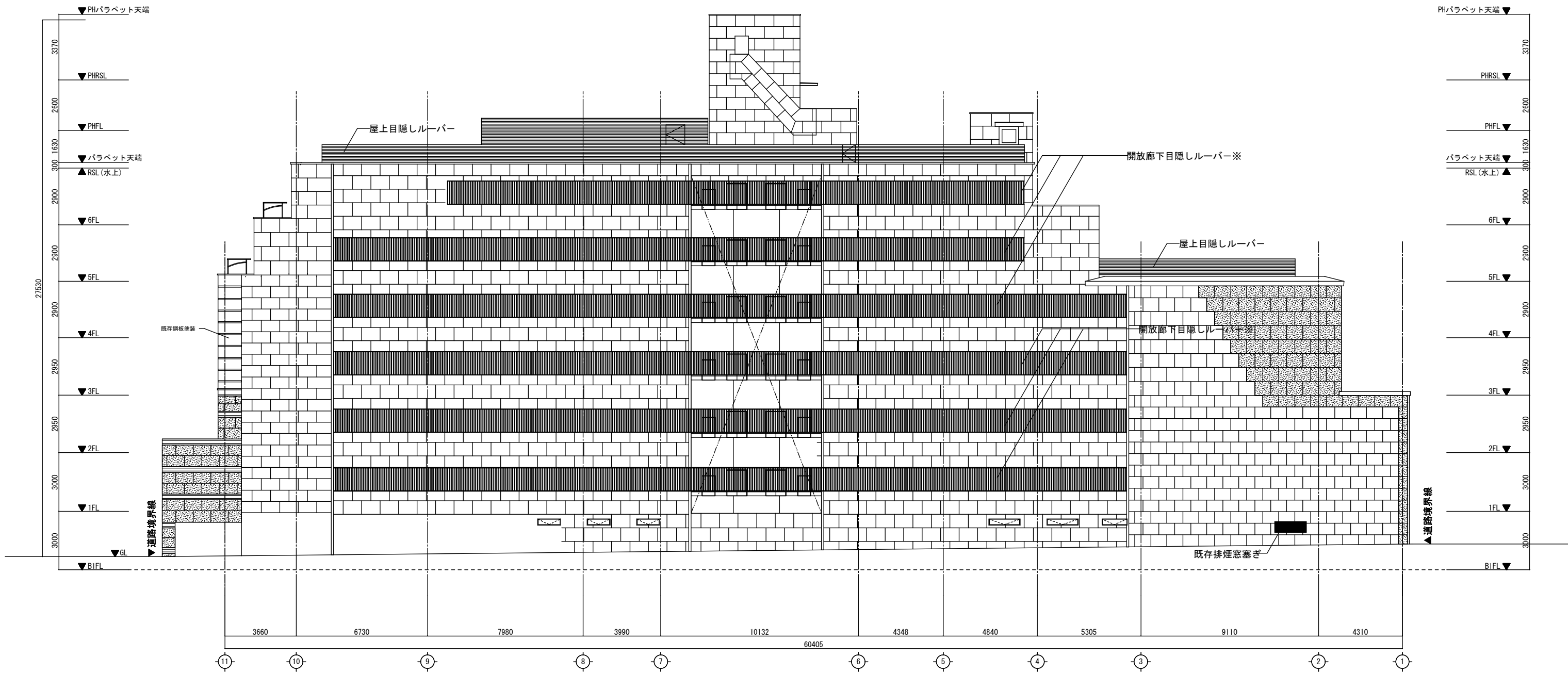
西立面図
